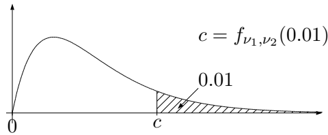
付表.8 エフ分布表 4 . W \sim F_{\nu_1, \nu_2} の時の , P(W > c) = 0.01 となる c の表
