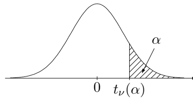
自由度 \nu のティー分布 t_\nu
