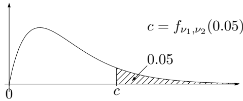
付表.6 エフ分布表 2 . W \sim F_{\nu_1, \nu_2} の時の , P(W > c) = 0.05 となる c の表
