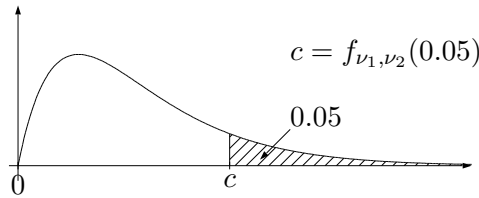
付表.5 エフ分布表 1 . W \sim F_{\nu_1, \nu_2} の時の , P(W > c) = 0.05 となる c の表
