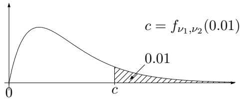
付表.7 エフ分布表 3 . W \sim F_{\nu_1, \nu_2} の時の , P(W > c) = 0.01 となる c の表
