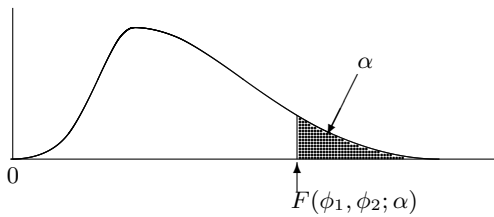
付表 4.1 F 分布表 (上側 5% 点) F(\phi_1, \phi_2; 0.05)
